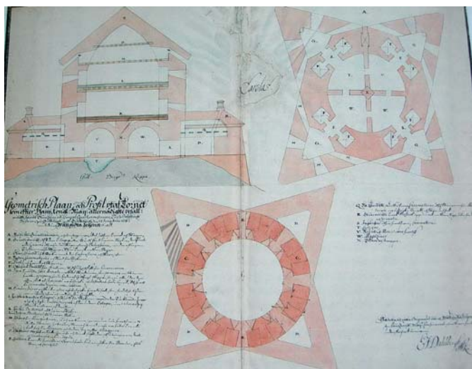
Planritning över Skansen Lejonet av Erik Dahlbergh
